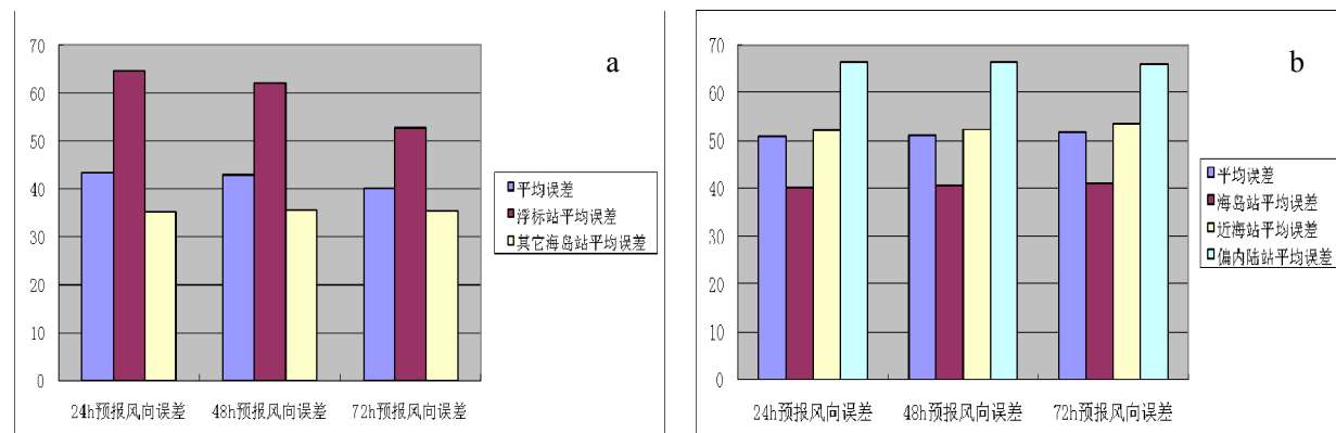
图 8(a) 沿海代表站风向绝对误差
