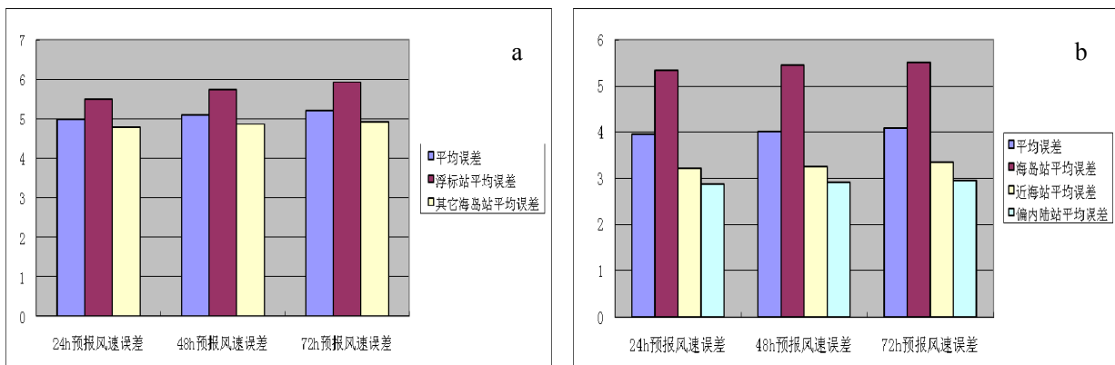
图7(a) 沿海代表站风速绝对误差
