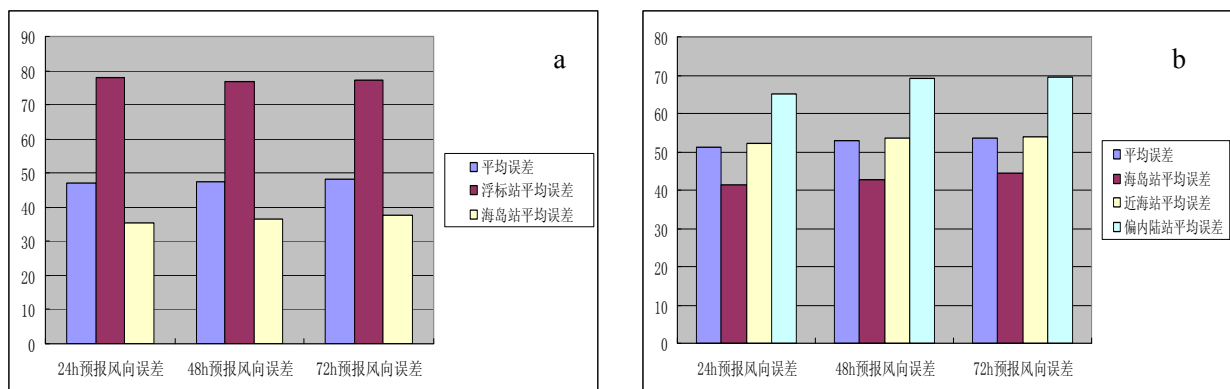
图 6(a) 沿海代表站风向绝对误差
