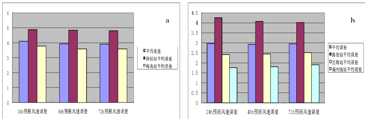
图 5(a) 沿海代表站风速绝对误差
