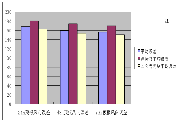
图 10(a) 沿海代表站风向绝对误差
