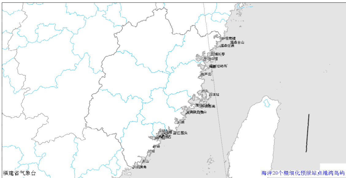
图3 港湾岛屿26个预报质量评定站
