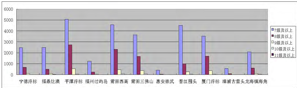
图2 2011-2012年冬半年福建省沿海地区11个预报质量评定代表站的极大风力分布图
