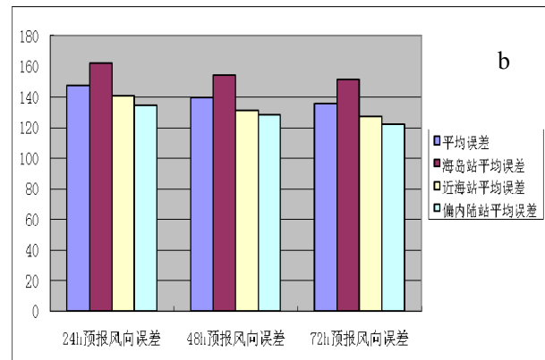
(b) 港湾岛屿代表站风向绝对误差
