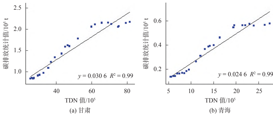
图 3 1995—2019 年甘肃 (a) 和青海 (b) 碳排放统计值 ( 10^5 t) 与 TDN 值 ( 10^5 ) 拟合结果
