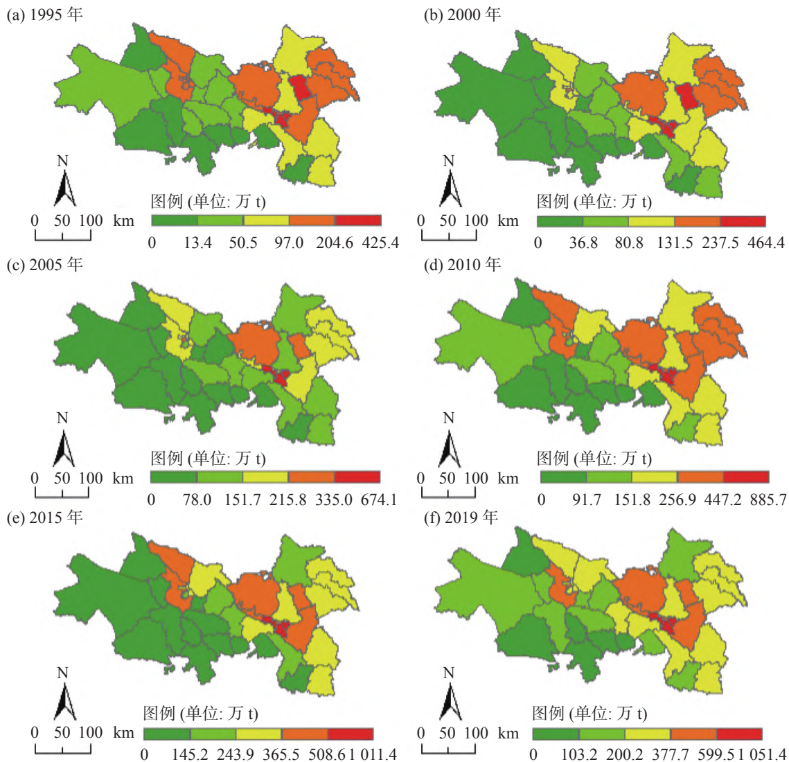
图6 1995—2019年兰西城市群县级碳排放量空间分布
