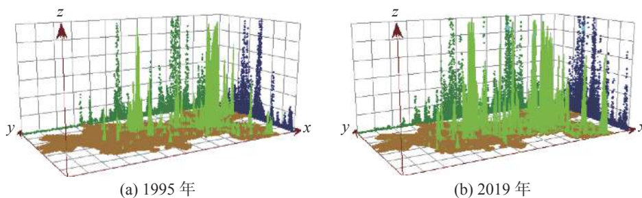
图9 1995年和2019年兰西城市群栅格尺度碳排放空间分布趋势
