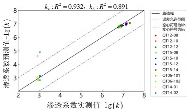
图 5 XGB 模型预测值-实测值对比图
