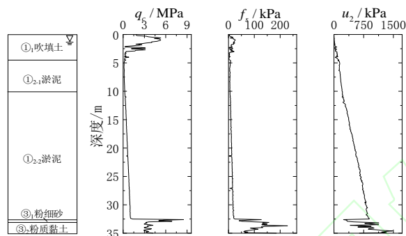
(a) 土层划分图 (b) 静力触探曲线图
