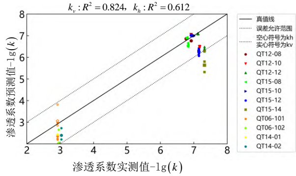
图 8 BPNN 模型预测值-实测值对比图
