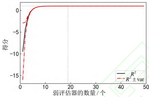
图2 训练集学习曲线图
